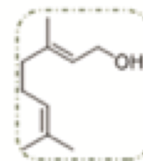
Geraniol
