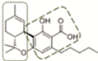
THCA
