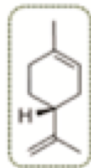
Limonene
